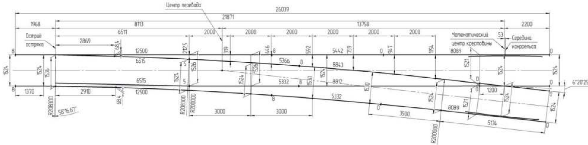
Схема геометрических размеров стрелочного перевода типа Р65 марки 1/9 колеи 1524 мм пр. ЛПТП.665121.102Кz; (-01)
