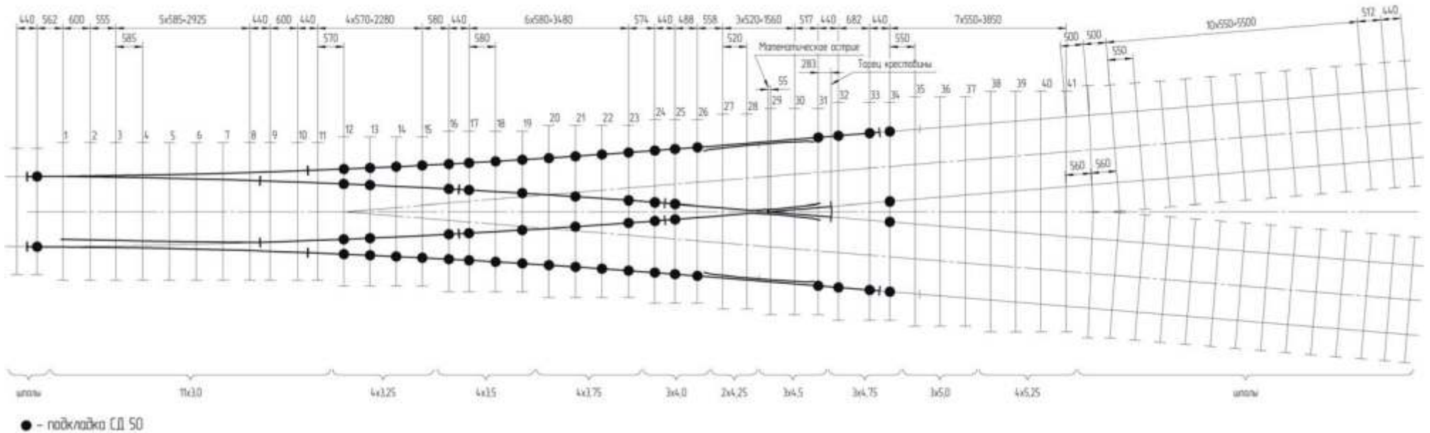
Схема укладки стрелочного перевода симметричного типа P50 марки 1/6 пр. Kz1581.00.000
