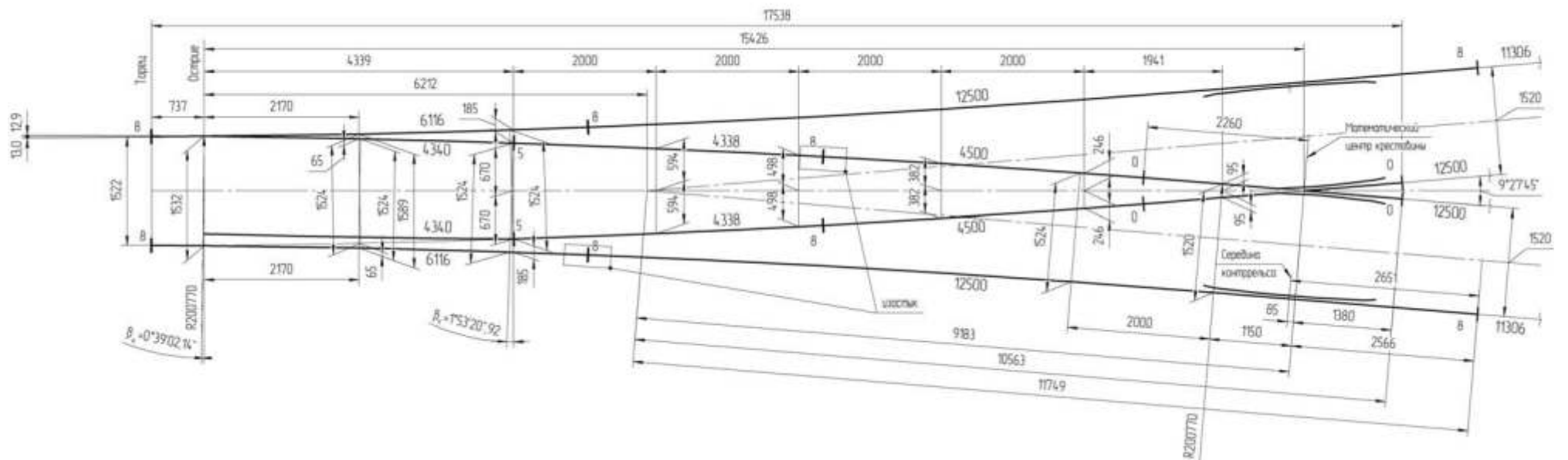
Схема геометрических размеров стрелочного перевода симметричного типа P50 марки 1/6 пр. Kz1581.00.000
