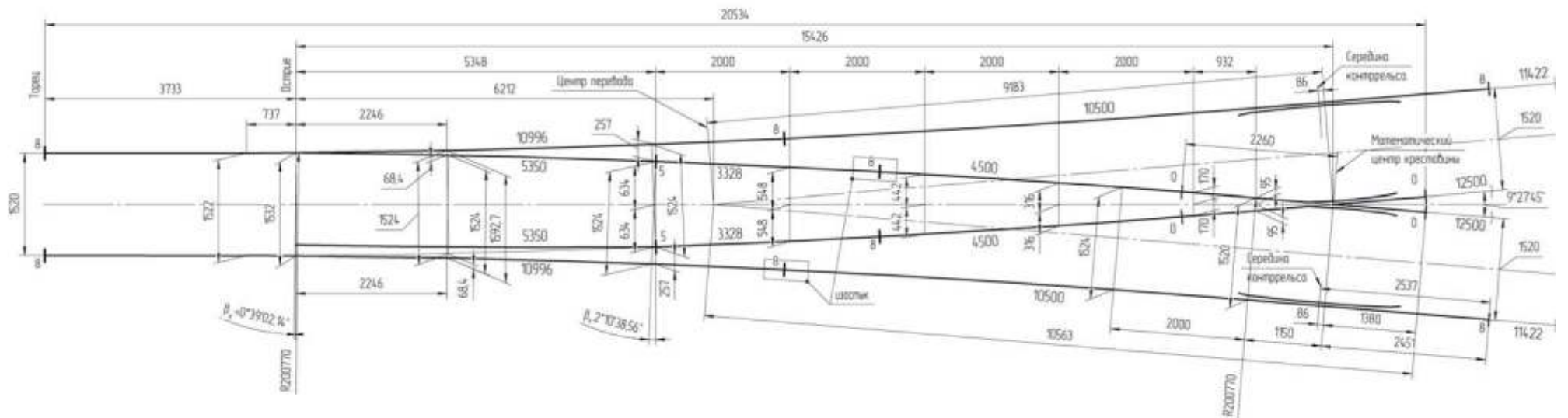
Схема геометрических размеров стрелочного перевода симметричного типа Р65 марки 1/6 пр. Kz2307.00.000-01
