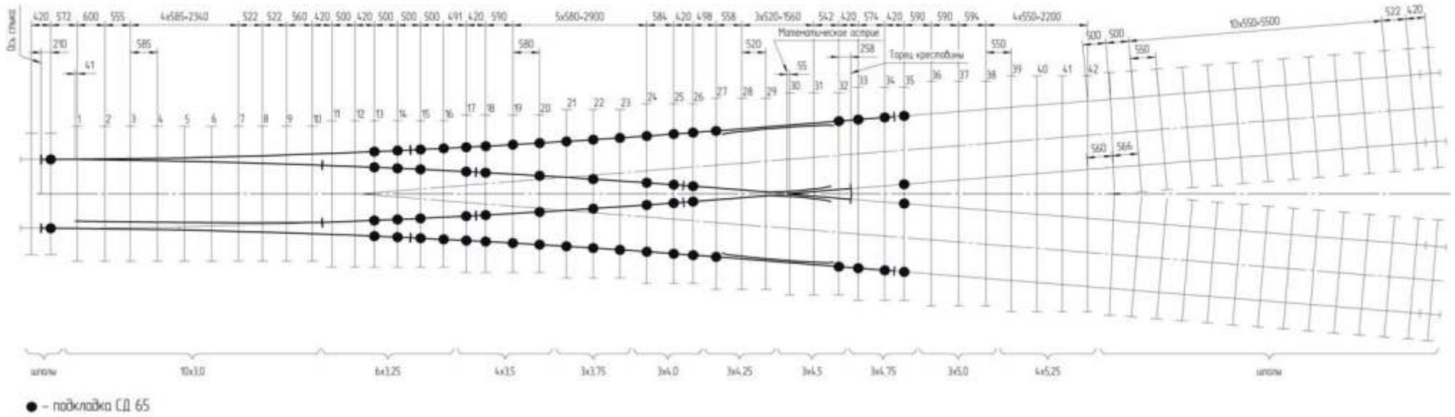
Схема геометрических размеров стрелочного перевода симметричного типа Р65 марки 1/6 пр. Kz2307.00.000
