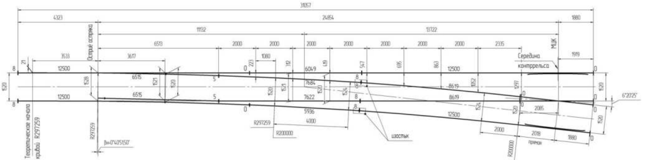
Схема геометрических размеров стрелочного перевода типа P50 марки 1/9 пр. Kz2643.00.000; (-01)
