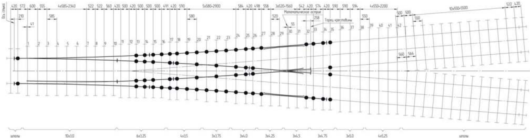
Схема укладки стрелочного перевода симметричного типа Р65 марки 1/6 пр. Kz2307.00.000
