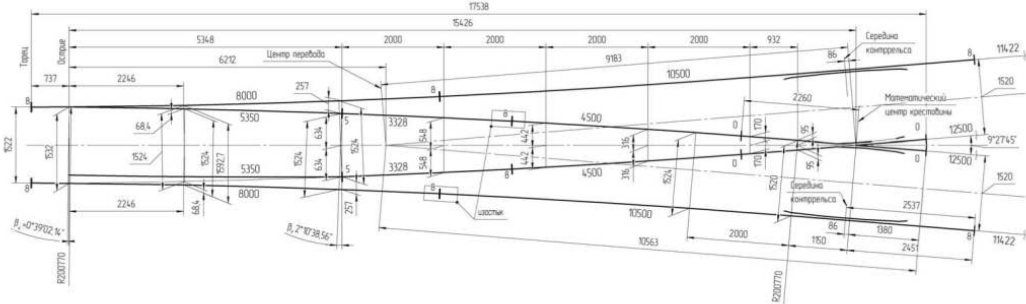
Схема геометрических размеров стрелочного перевода симметричного типа Р65 марки 1/6 пр. Kz2307.00.000
