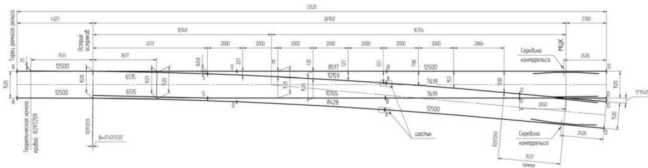
Схема геометрических размеров стрелочного перевода типа P50 марки 1/11 пр. Kz2642.00.000; (-01)
