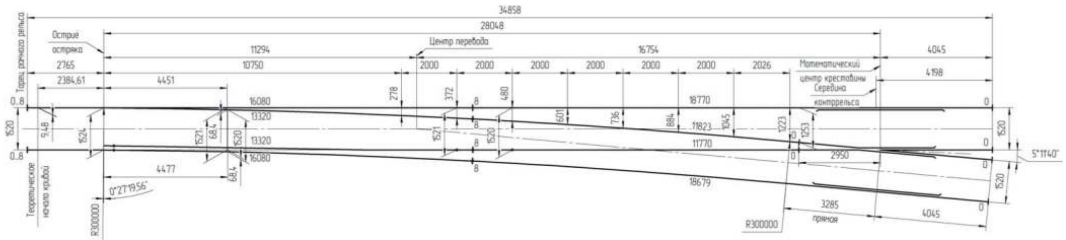
Схема геометрических размеров стрелочного перевода типа Р65 марки 1/11 на ж.д. брусьях пр. Кz2750.00.000-02; (-03; -04; -05)
